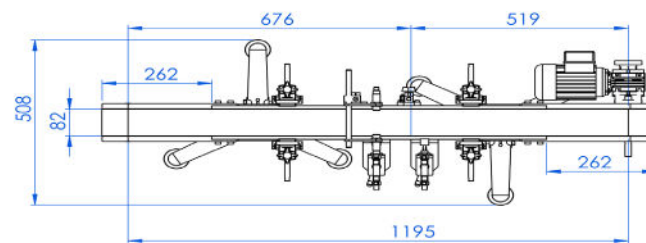
Convoyeur indépendant 1 éclusage
