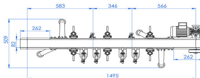
Convoyeur indépendant 2 éclusages
